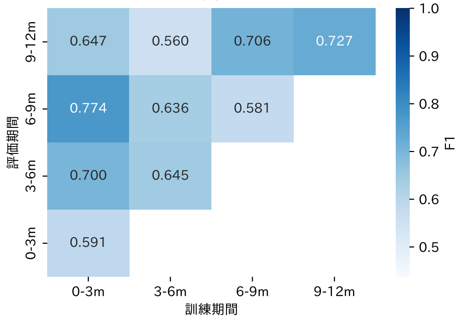
F1
