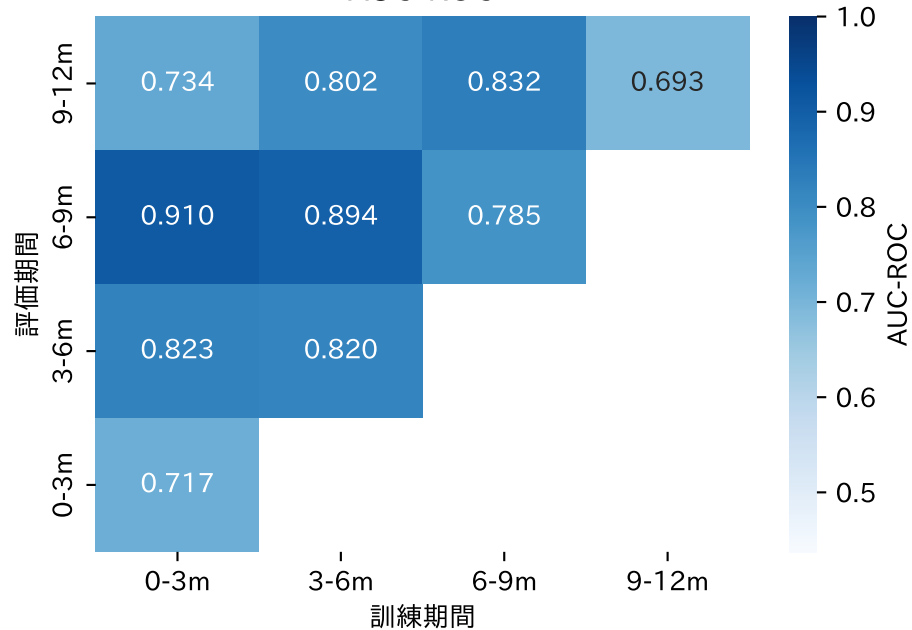
AUC-ROC
