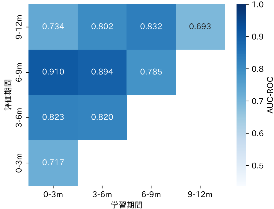
AUC-ROC
