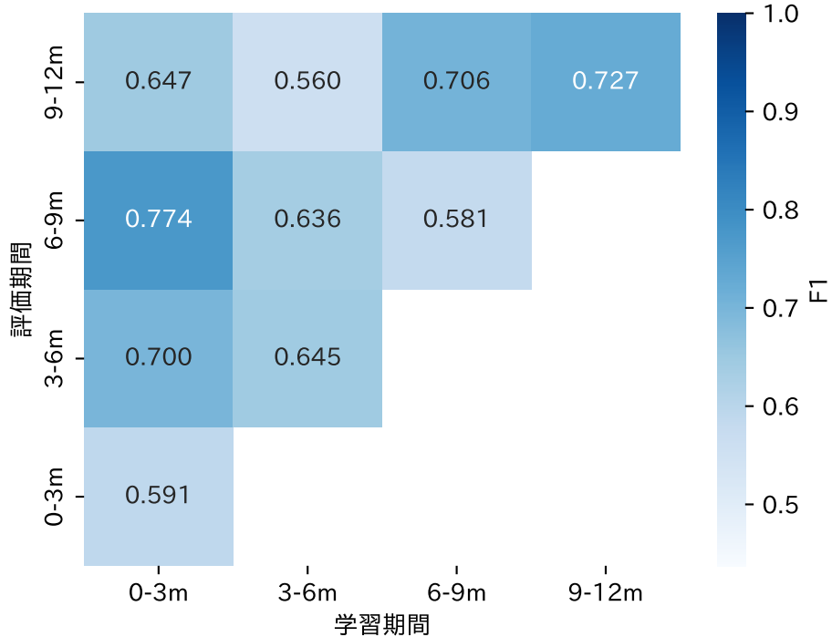
F1
