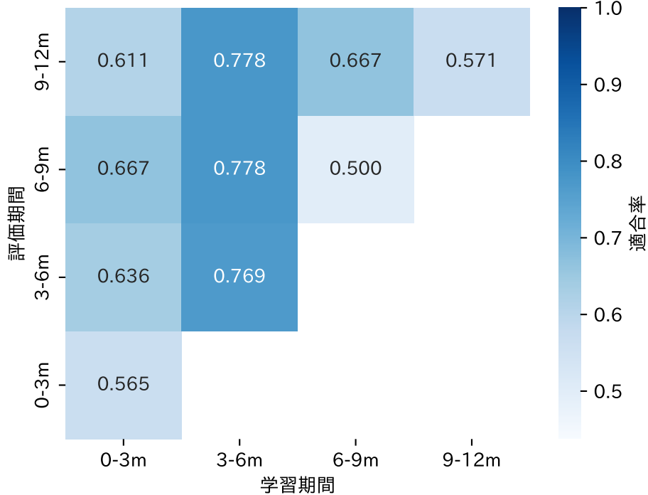
F1
