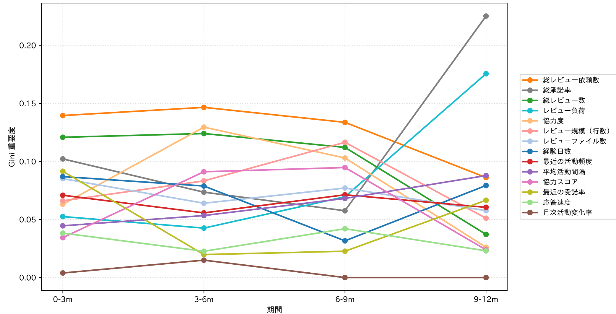
RF: 特徴量重要度 (期間別, Gini)
