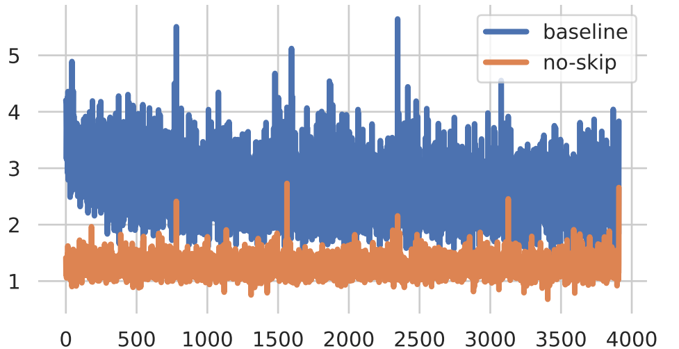
Gradient Norm
