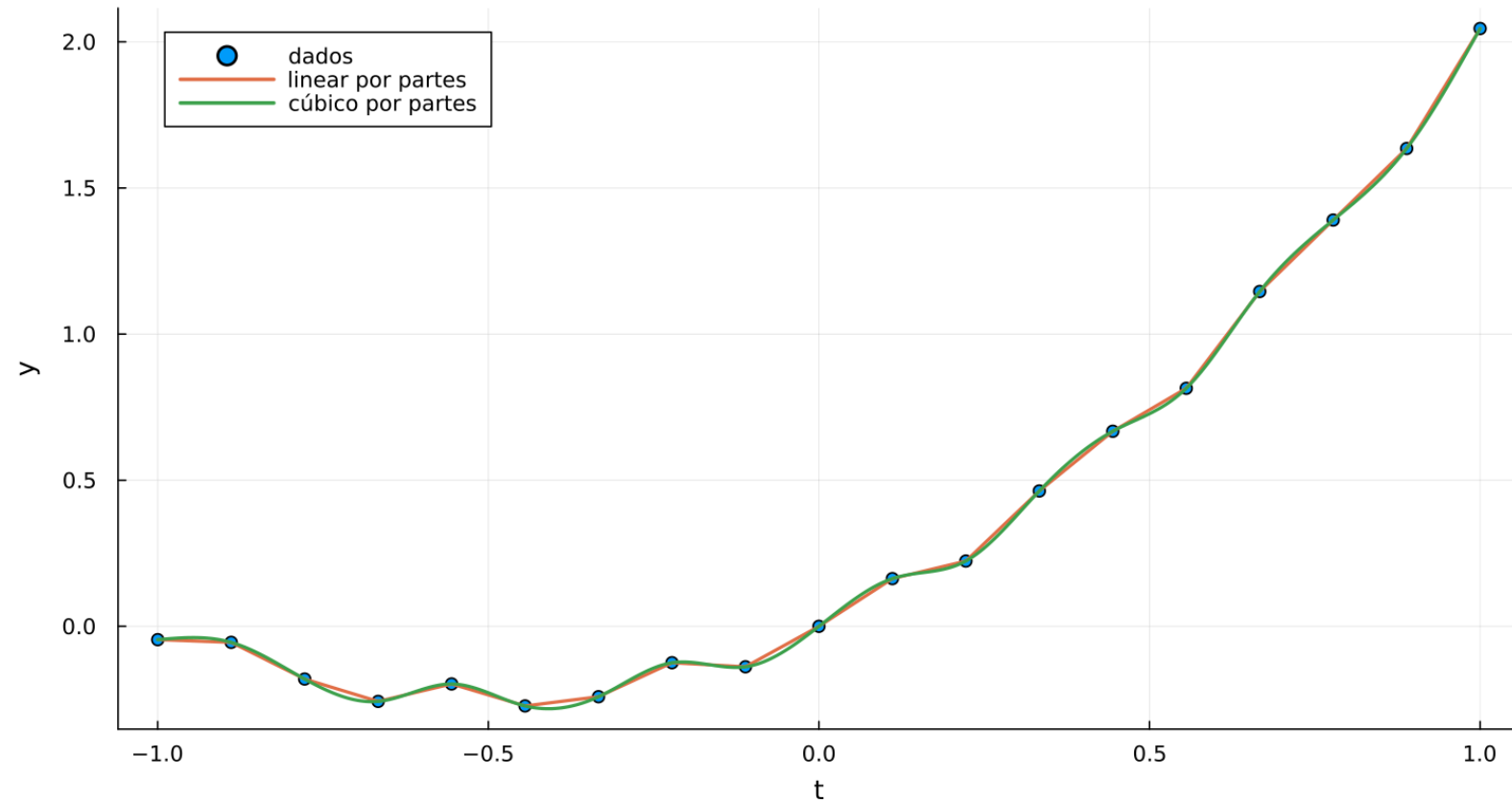
Polinômios por partes, n = 18
