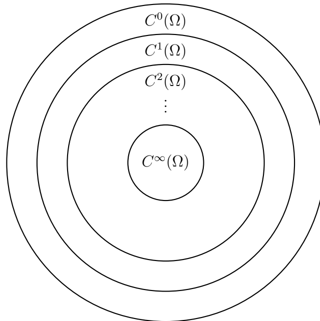
Abbildung 2: Schematische Darstellung der Hierarchie C^\infty(\Omega) \subset \dots \subset C^2(\Omega) \subset C^1(\Omega) \subset C^0(\Omega) . Je höher die Regularität, desto kleiner der entsprechende Funktionenraum.
