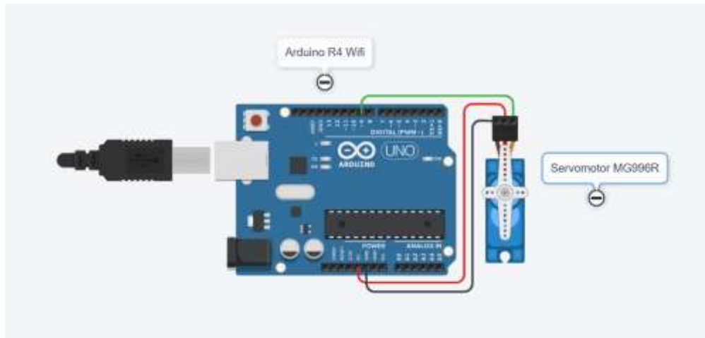
Figura 1. Diagrama de conexiones (Tinkercad Circuits).
