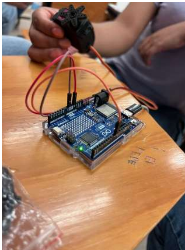
Figura 5. Armado físico con el Arduino UNO R4 WiFi y el servomotor MG996R.
