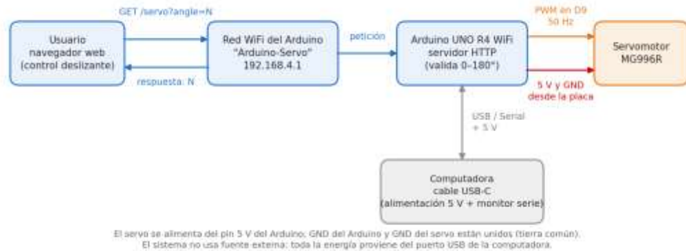
Figura 2. Diagrama de bloques del sistema.
