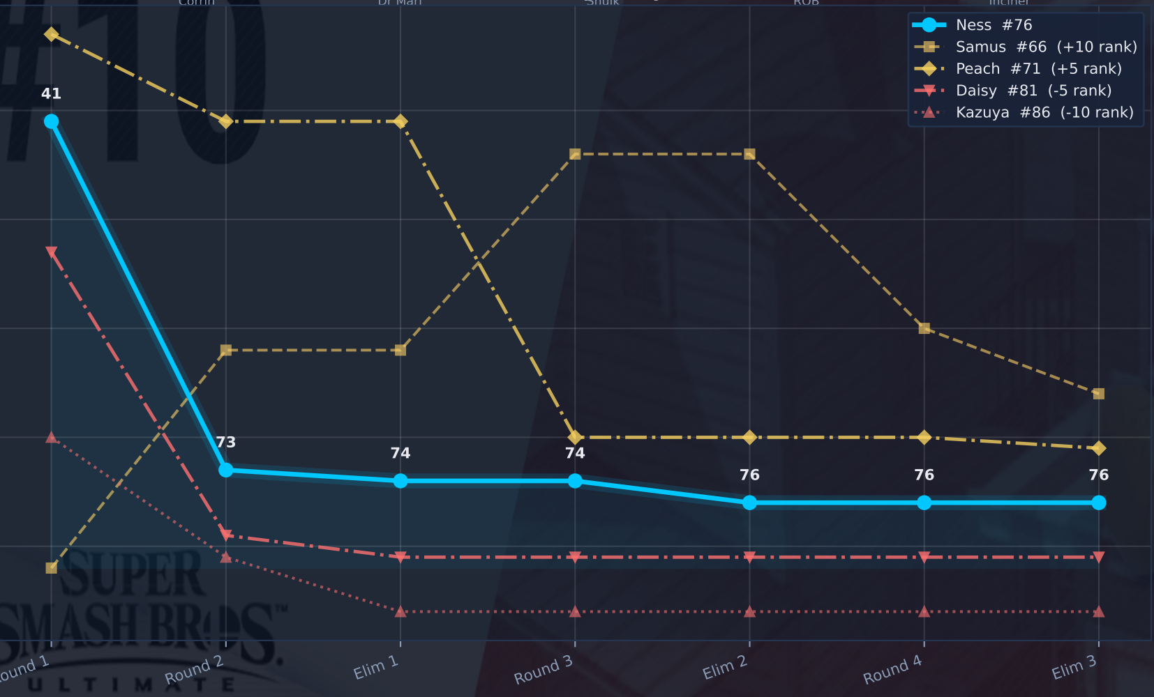
Rank Trajectory
