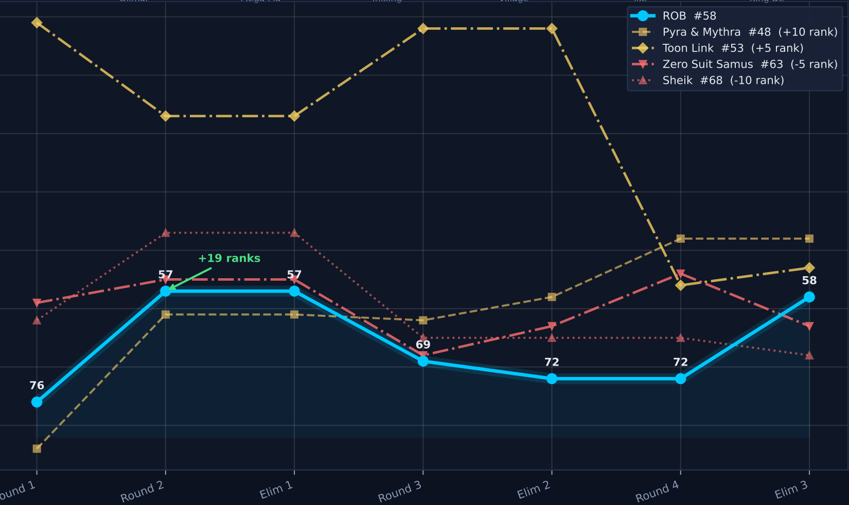
Rank Trajectory
