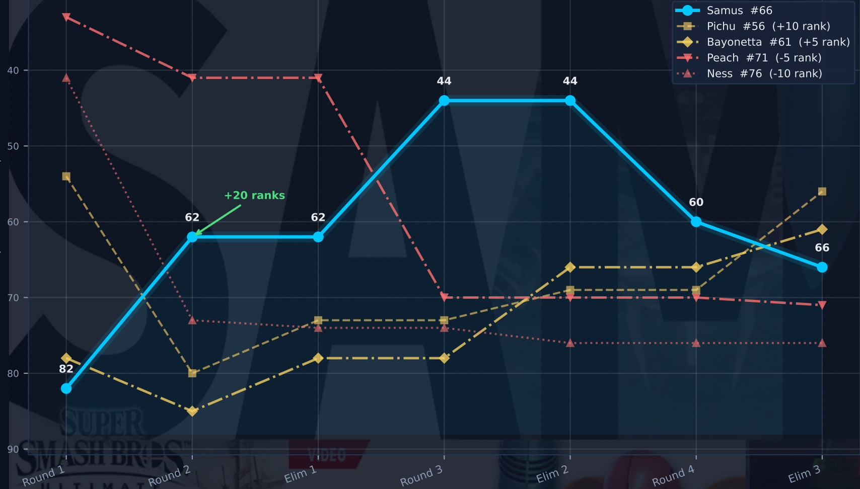
Rank Trajectory
