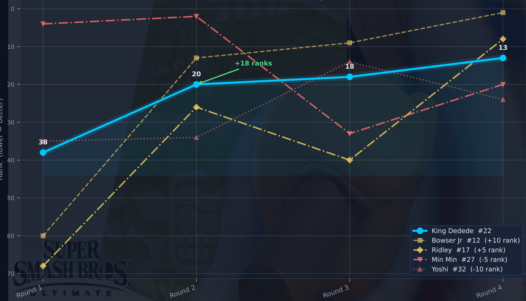
Rank Trajectory
