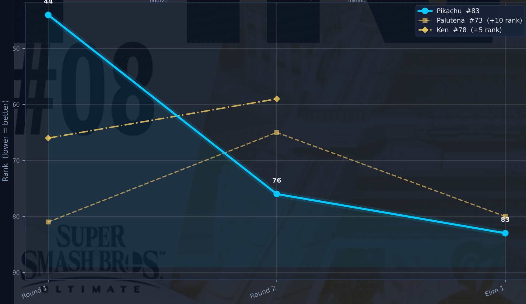
Rank Trajectory
