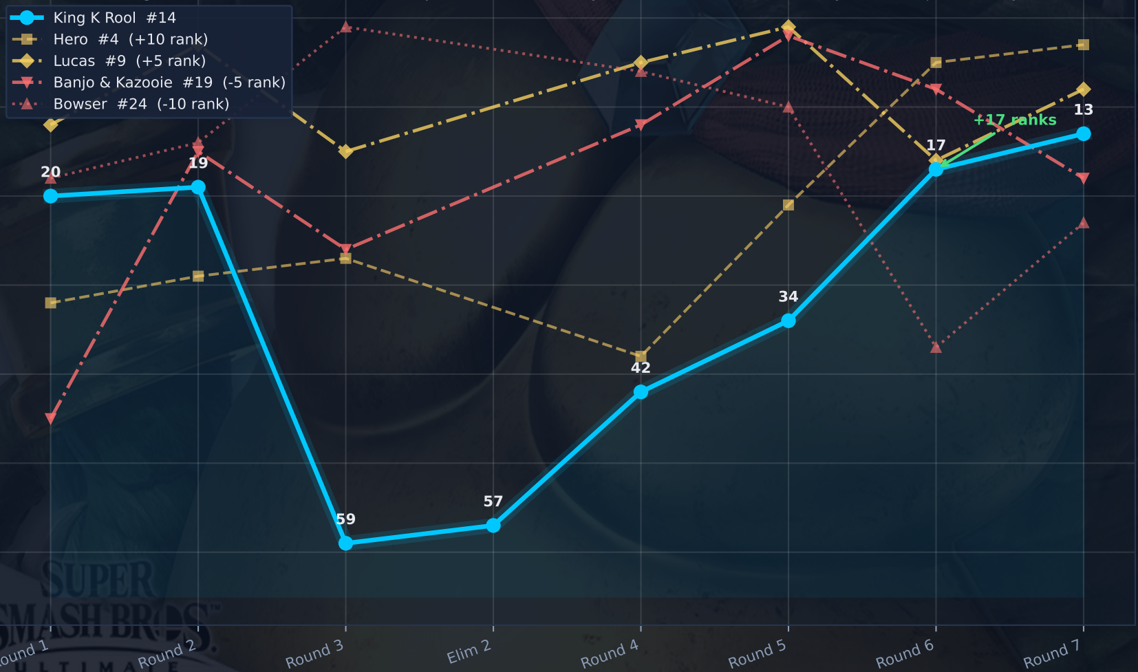
Rank Trajectory
