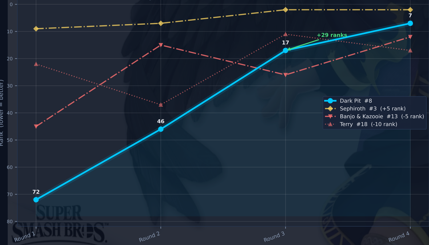
Rank Trajectory
