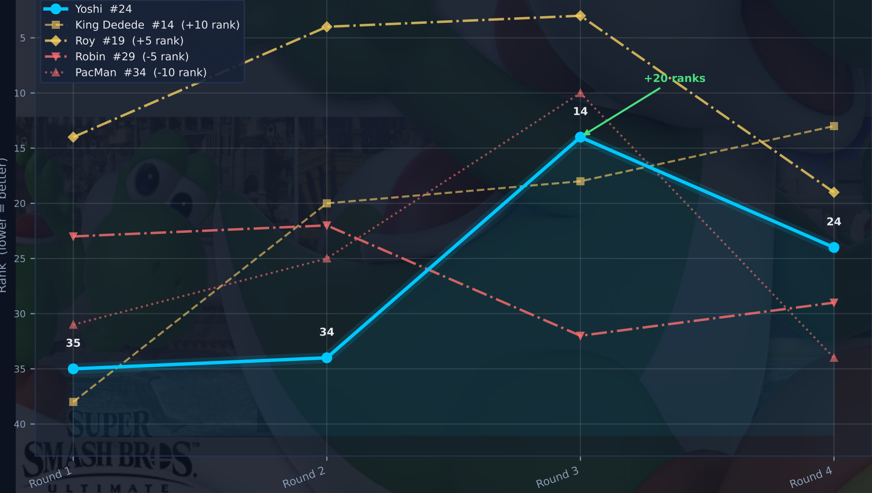
Rank Trajectory
