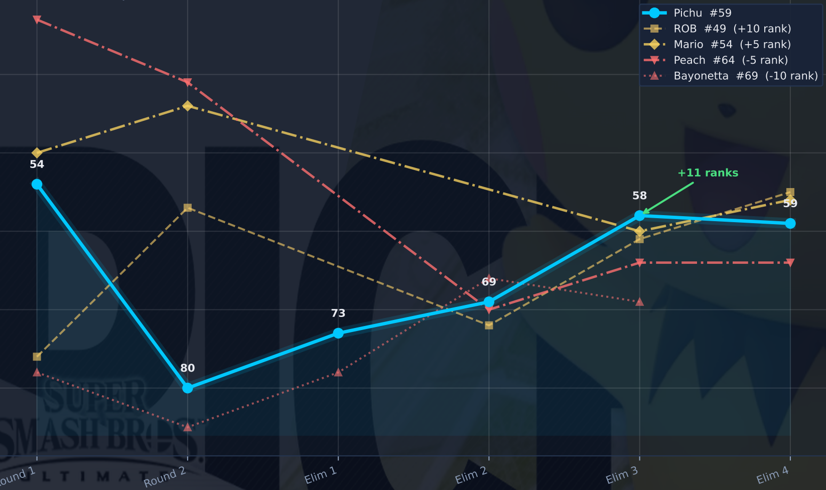
Rank Trajectory
