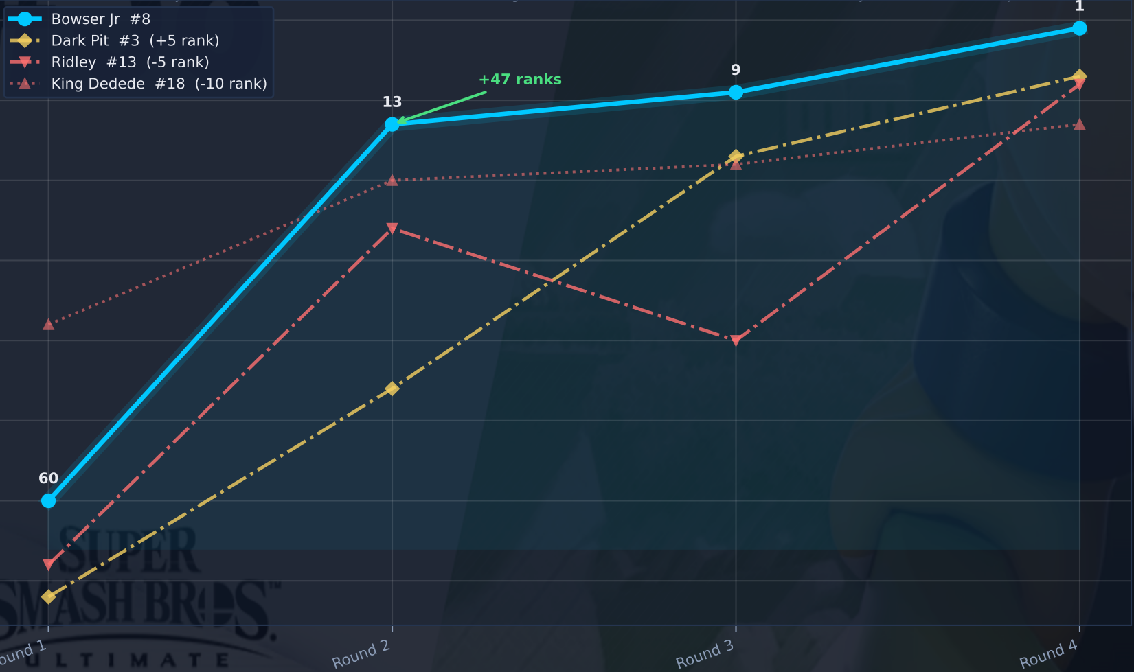
Rank Trajectory
