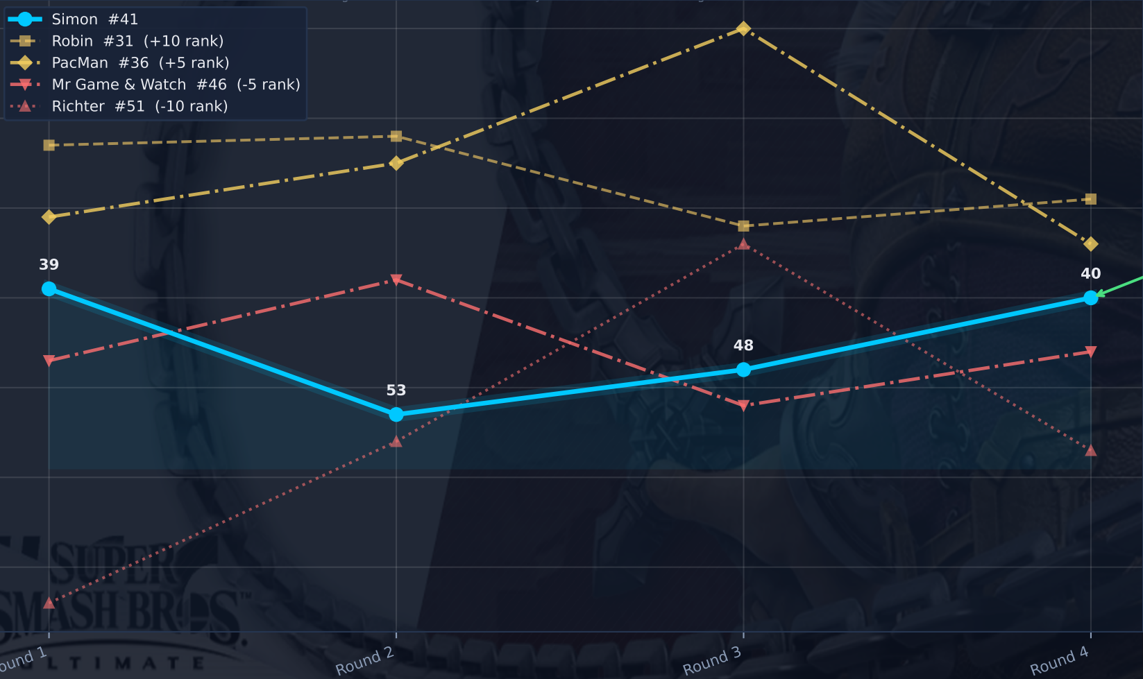
Rank Trajectory
