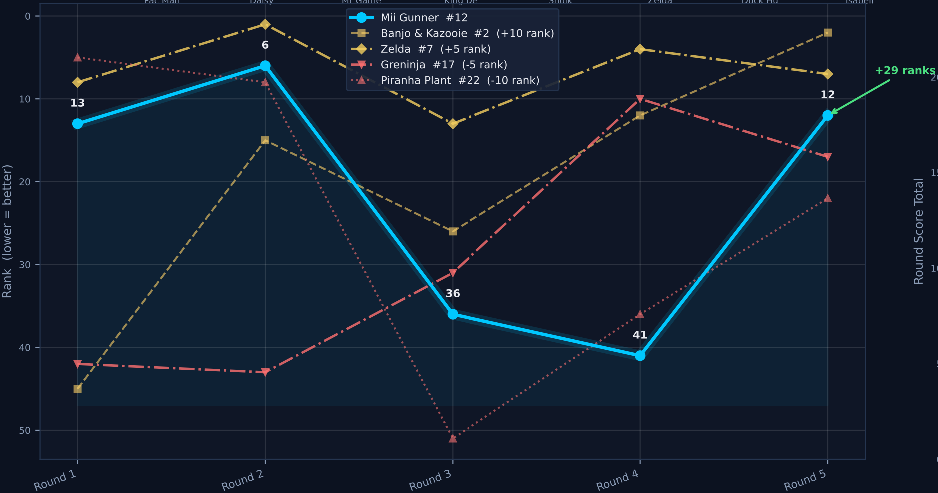
Rank Trajectory
