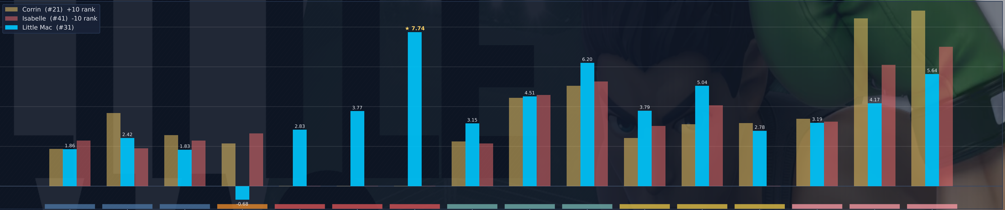
Rank Trajectory
