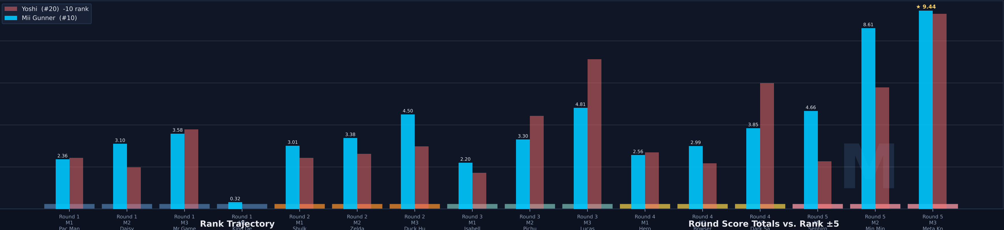
Rank Trajectory
