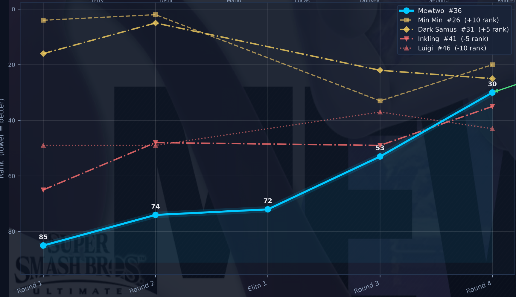
Rank Trajectory
