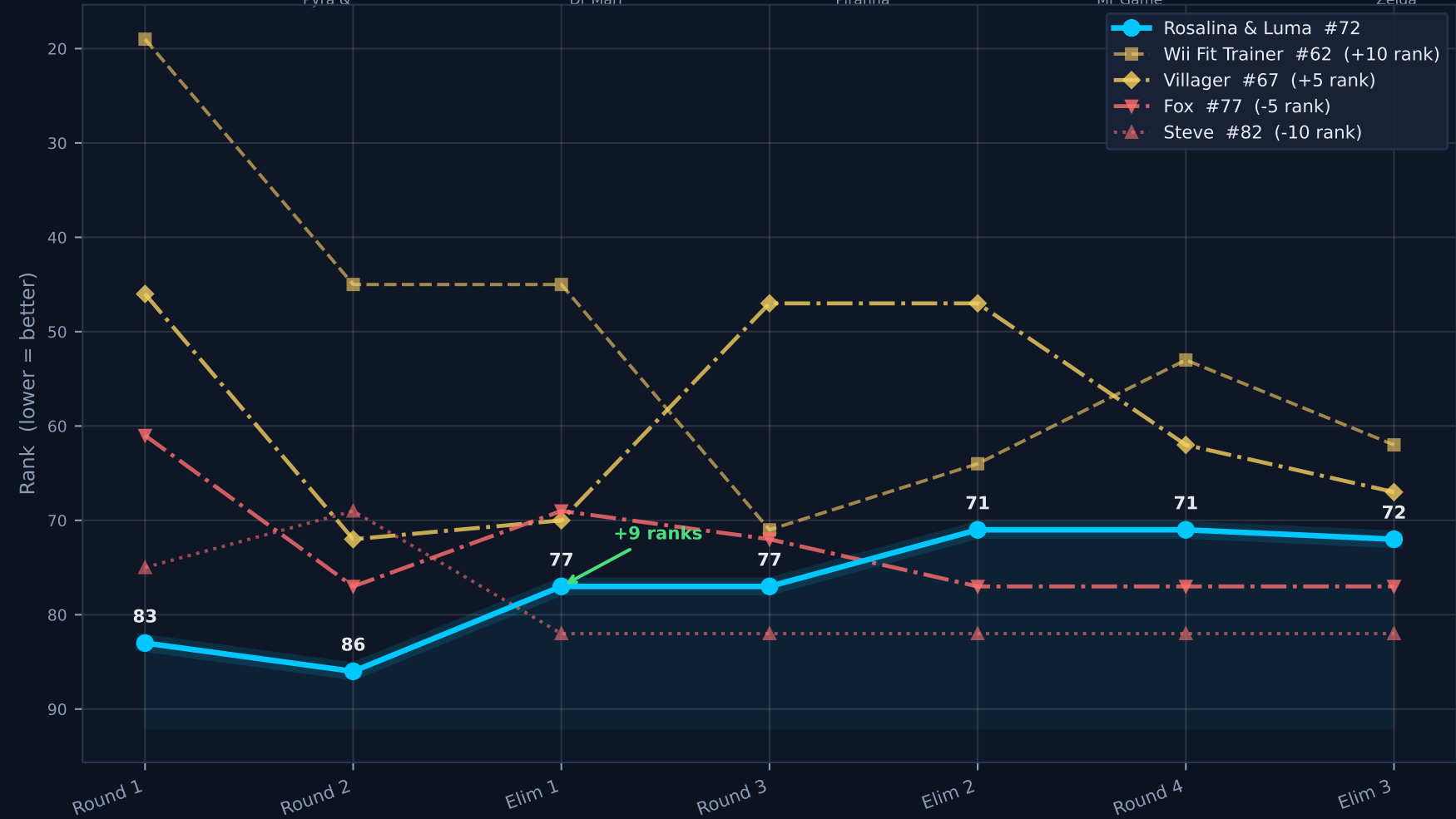
Rank Trajectory
