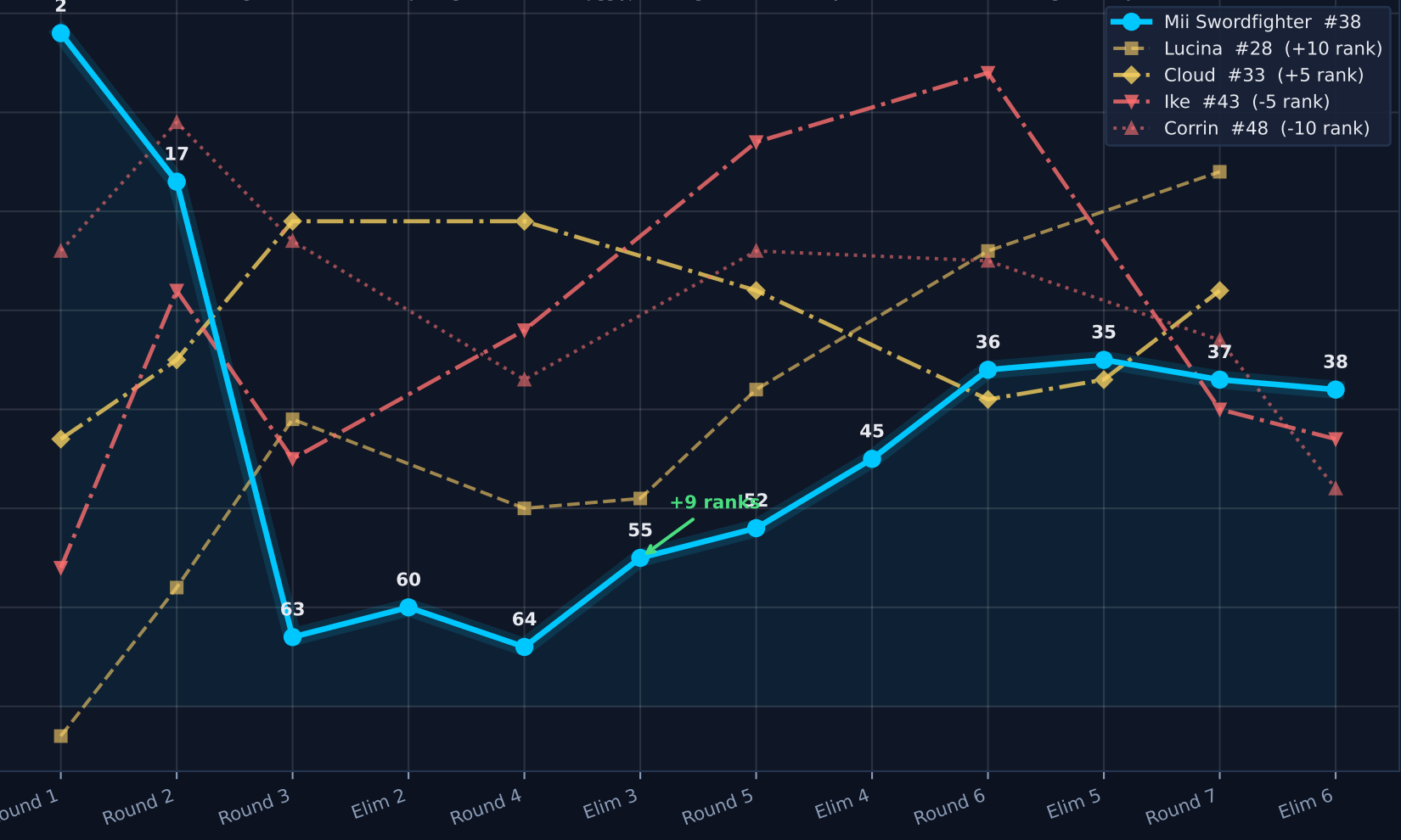
Rank Trajectory
