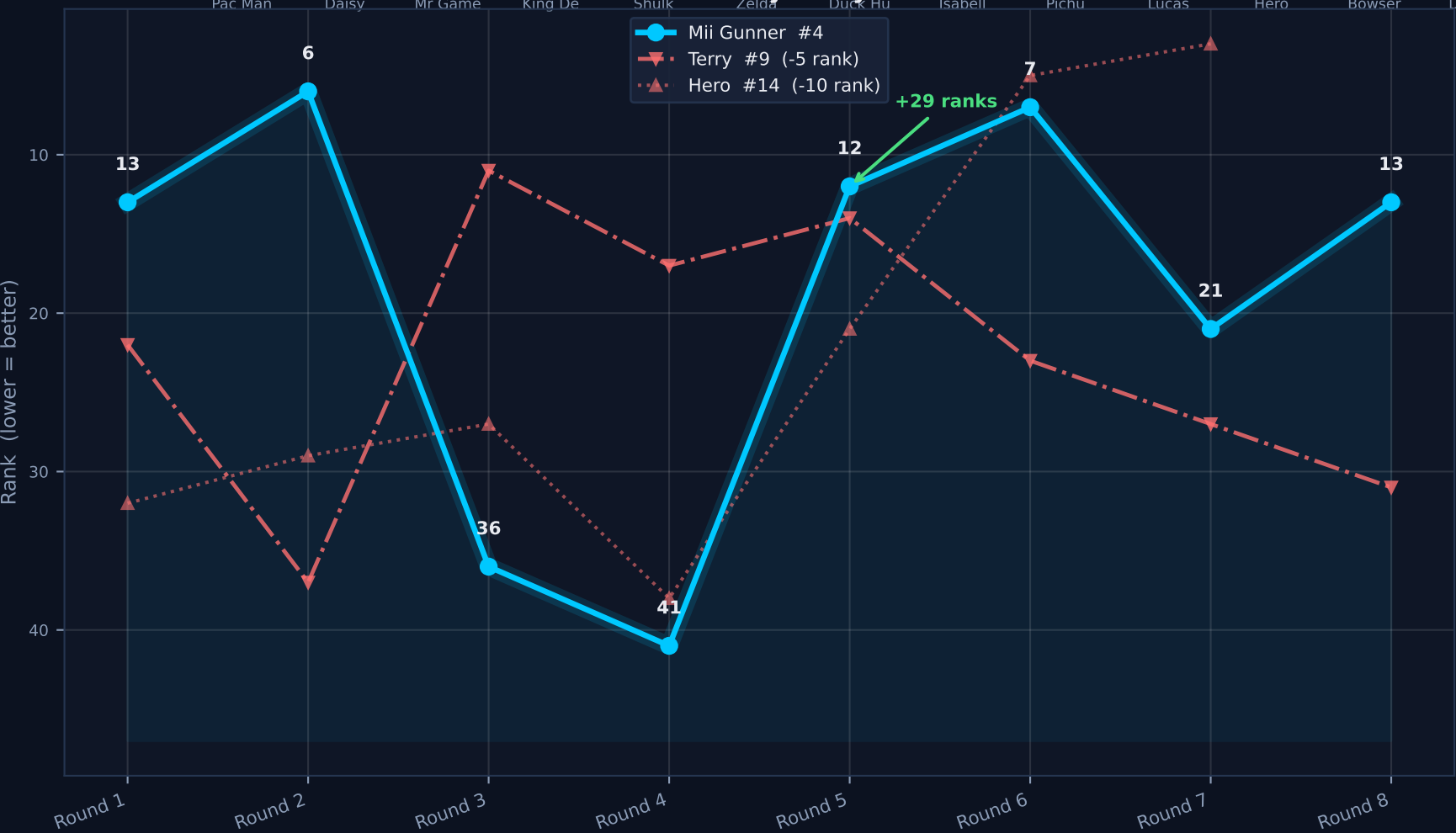
Rank Trajectory
