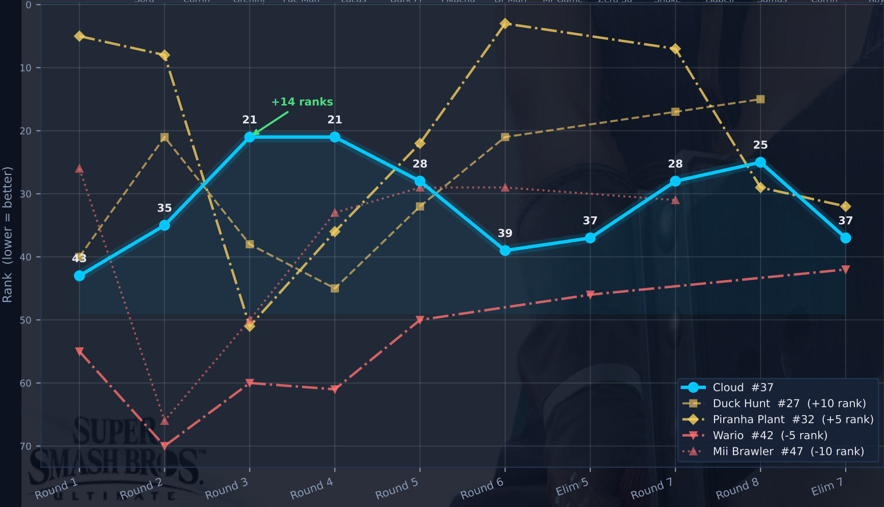
Rank Trajectory
