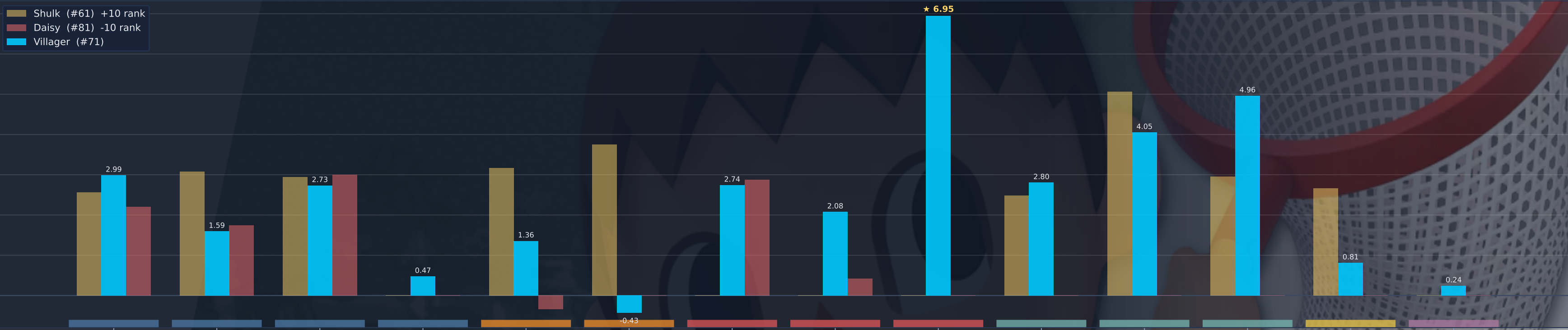
Rank Trajectory
