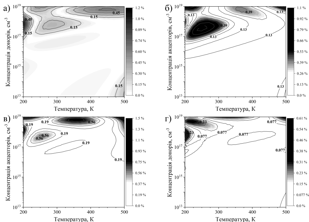
Рис. 2. Температурні та концентраційні залежності величини абсолютної відносної похибки при оцінці рухливості носіїв заряду у кремнії за допомогою виразів (12) – (15). Представлені випадки оцінки рухливості електронів (а, б) та дірок (в, г), коли вони є основними (а, в) та неосновними (б, г) носіями заряду.
