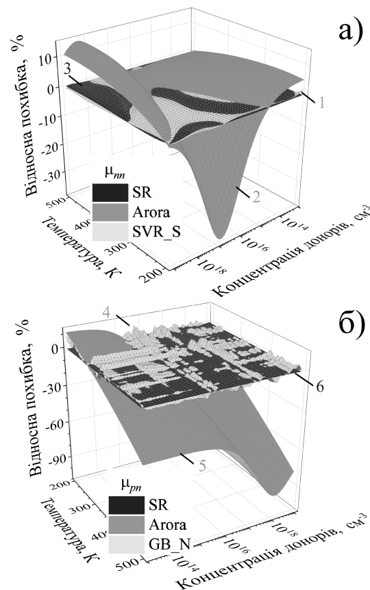
Рис. 4. Температурні та концентраційні залежності помилки розрахунків рухливості основних (а) та неосновних (б) носіїв за допомогою різних моделей відносно теорії Klaassen. Модель: SVR_S (поверхня 1), Arora (2, 5), SR (3, 6), GB_N (4).
