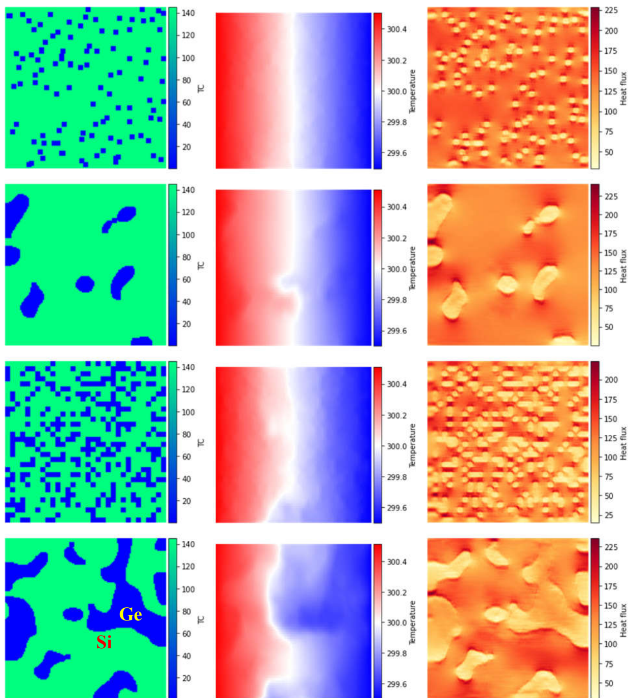
Рис.1. Вихідний розподіл фаз (лівий стовбець, зелене – кремній, синє - германій) та спрогнозовані розподіли температури (середній стовбець) і теплового потоку Q = \sqrt{Q_x^2 + Q_y^2} (правий стовбець). Частка германію становить 10% (перший та другий рядки) та 30% (третій та четвертий рядки), ступінь кластеризації 0 (перший та третій рядки) та 0,5 (другий та четвертий рядки).
