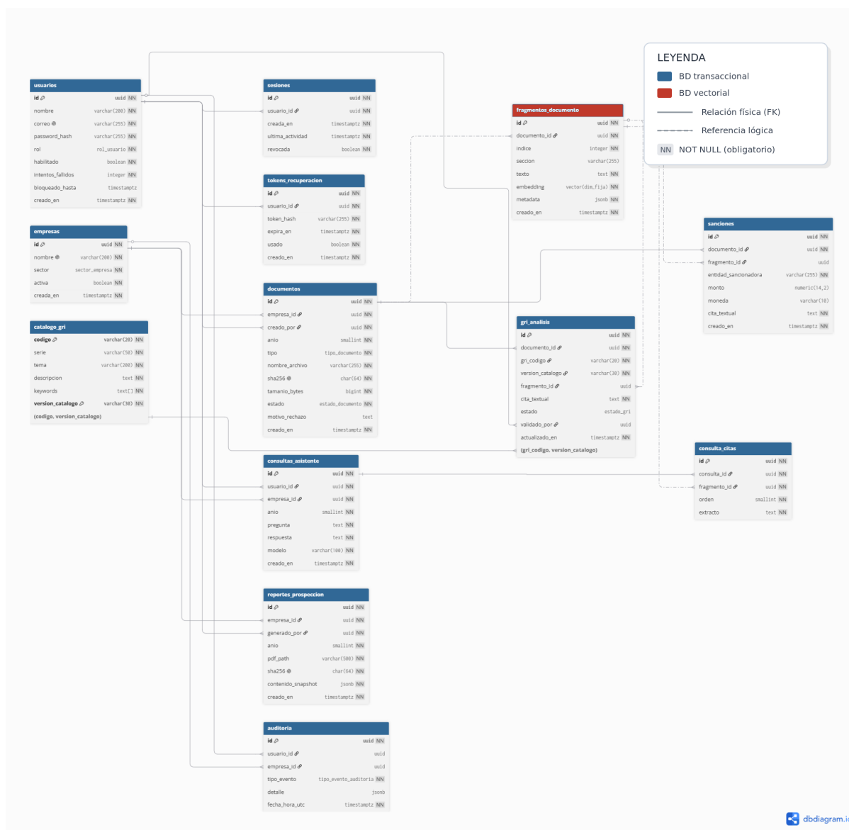
Modelo de datos de Iguallab
