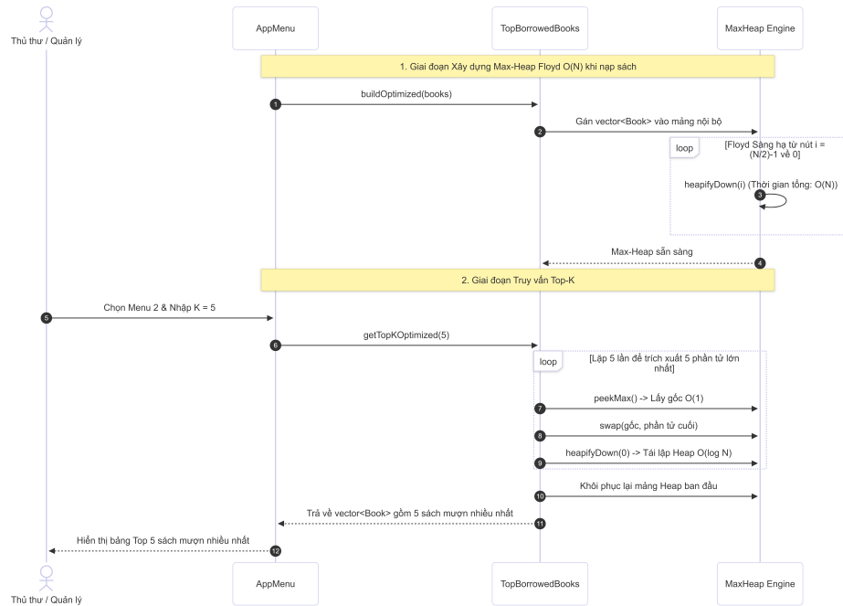
Hình 8. Sơ đồ tuần tự thể hiện luồng trích xuất sách mượn nhiều nhất (MC2)
