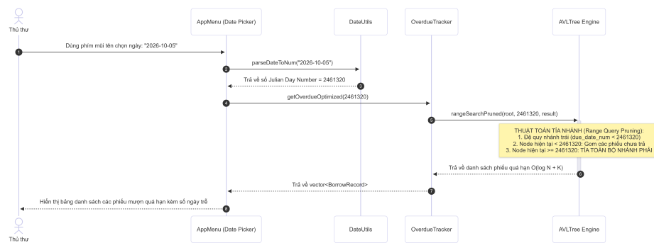
Hình 17. Sơ đồ tuần tự thể hiện luồng truy vết phiếu mượn quá hạn (RQ2)
