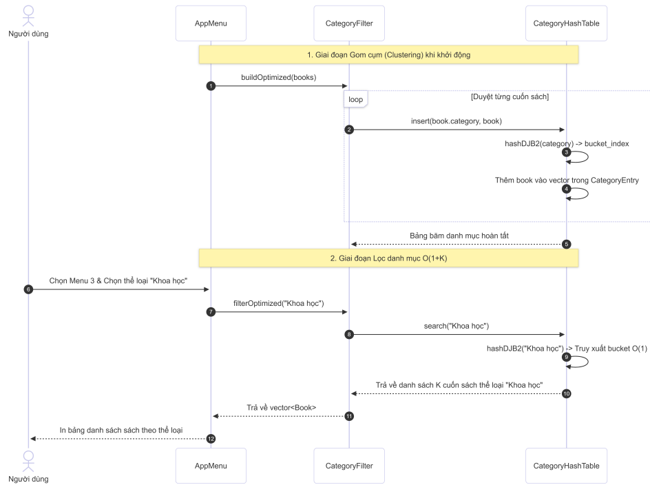
Hình 12. Sơ đồ tuần tự thể hiện luồng lọc sách theo thể loại (RQ1)
