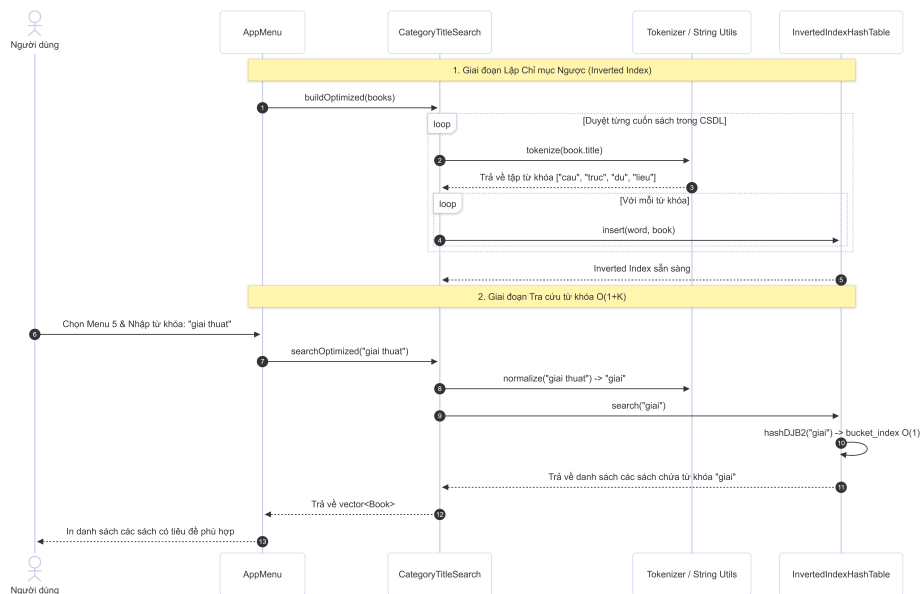
Hình 22. Sơ đồ tuần tự thể hiện luồng tìm kiếm tựa sách theo từ khóa (RQ3)
