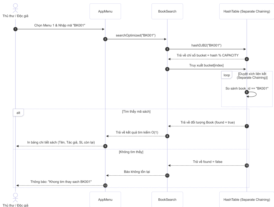
Hình 3. Sơ đồ tuần tự thể hiện luồng tra cứu sách theo mã định danh (MC1)
