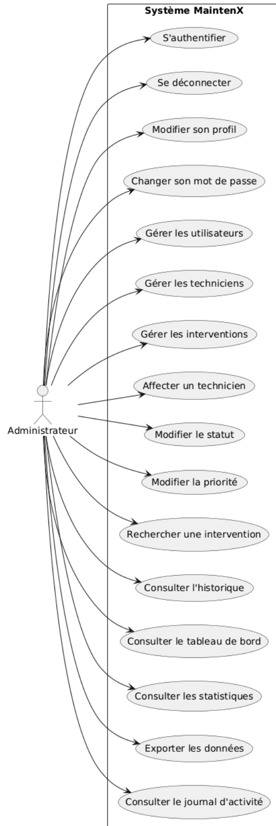
Figure 4 : Cas d'utilisation - Administrateur
