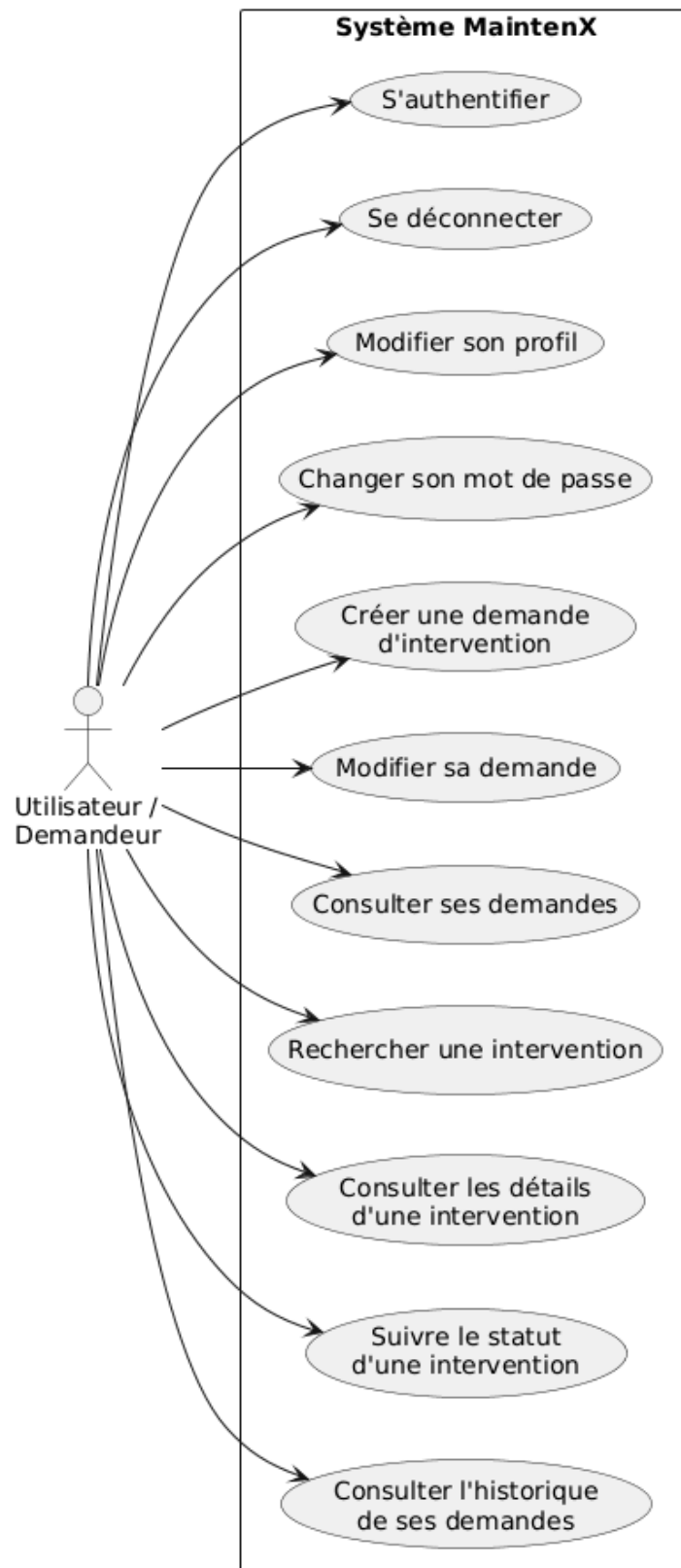
Figure 7 : Cas d'utilisation - Gestion des utilisateurs (détail)
