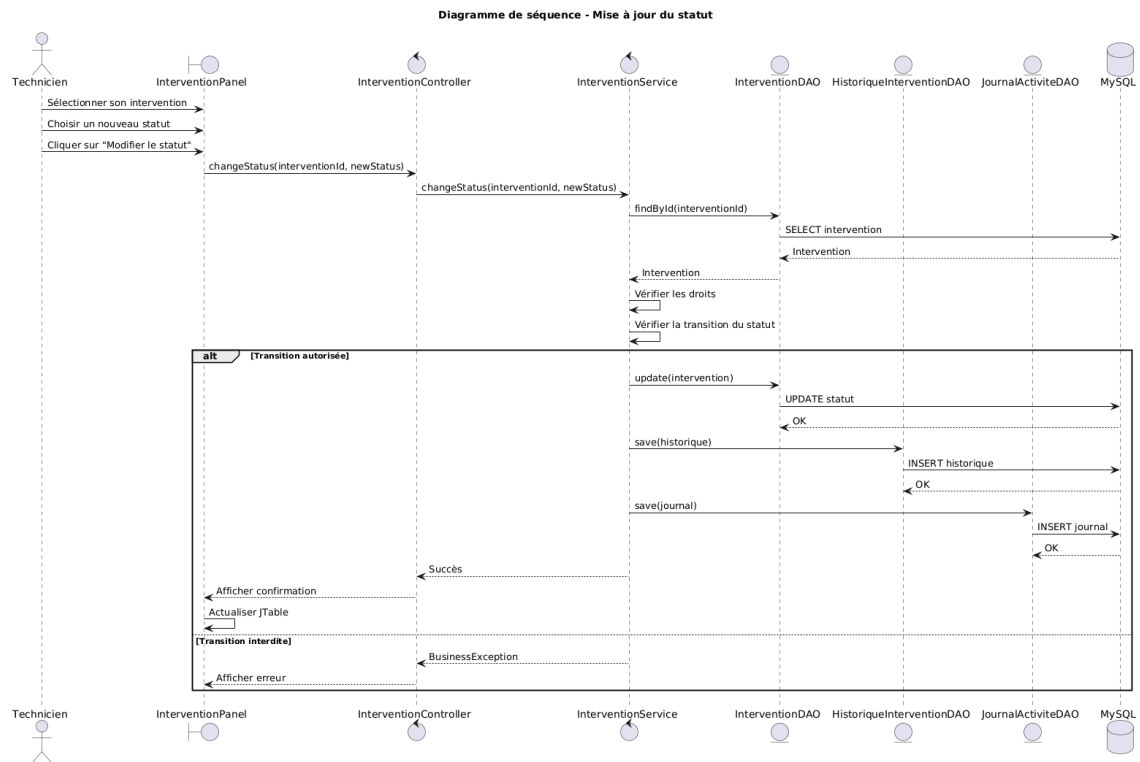
Figure 16 : Diagramme de séquence - Changement de statut
