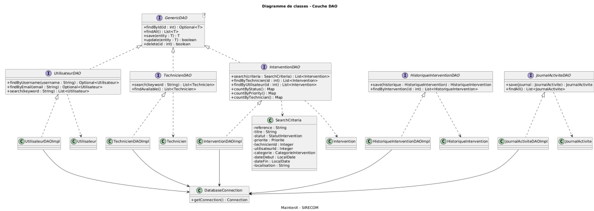
Figure 12 : Diagramme des classes DAO
