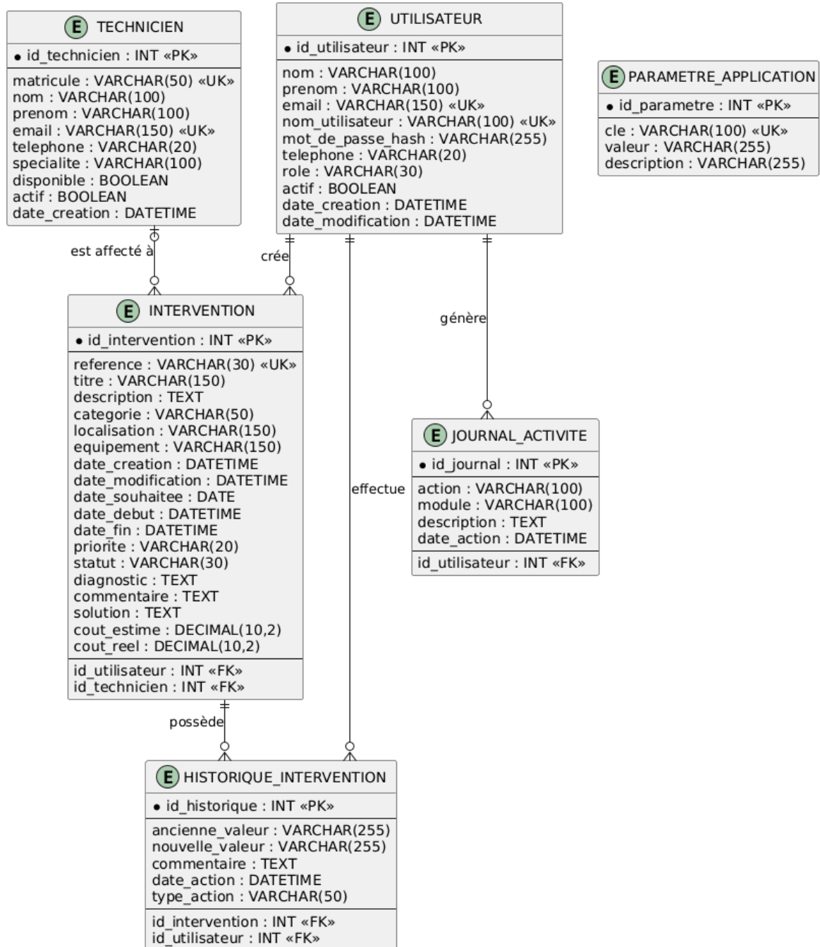
Figure 25 : Modèle Conceptuel de Données (MCD)
