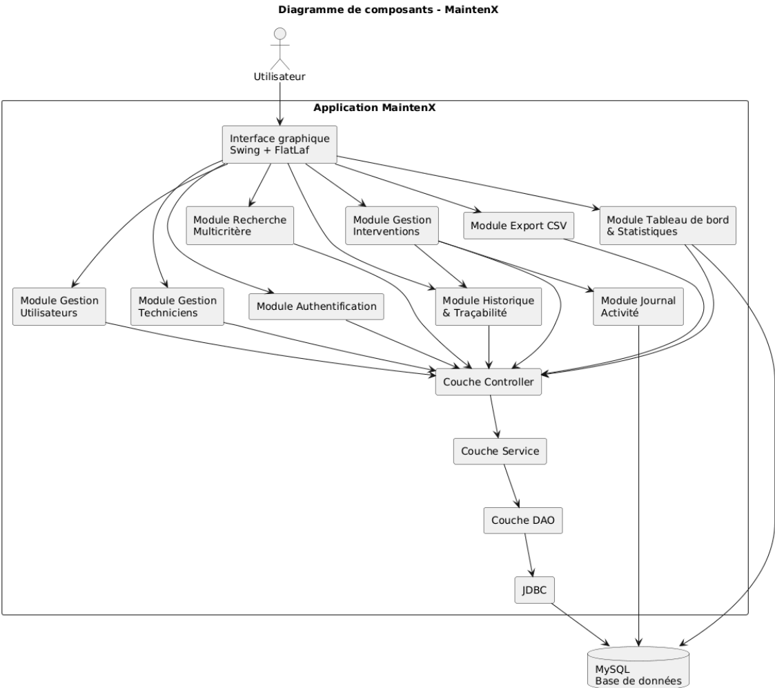
Application Java Swing de gestion de maintenance - SIRECOM
