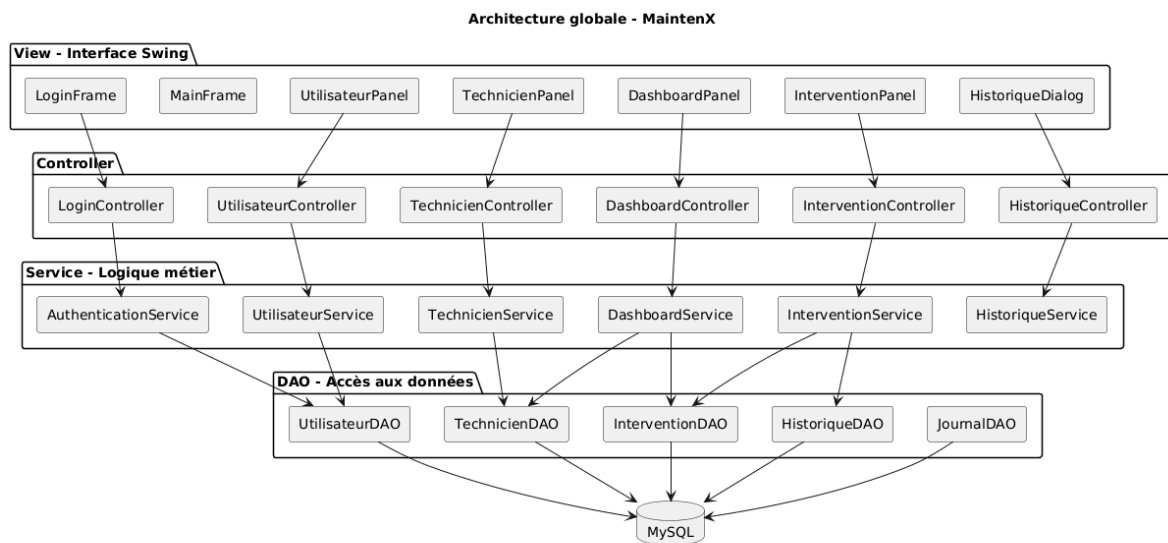
Application Java de gestion des interventions - SIRECOM
