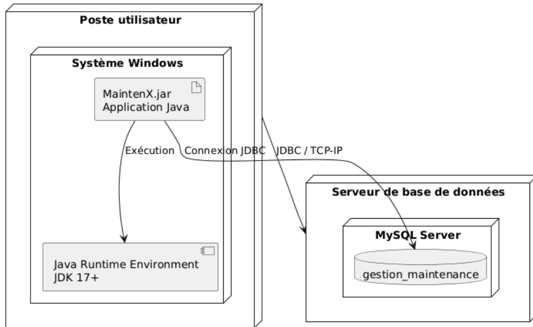
Figure 24 : Diagramme de déploiement
