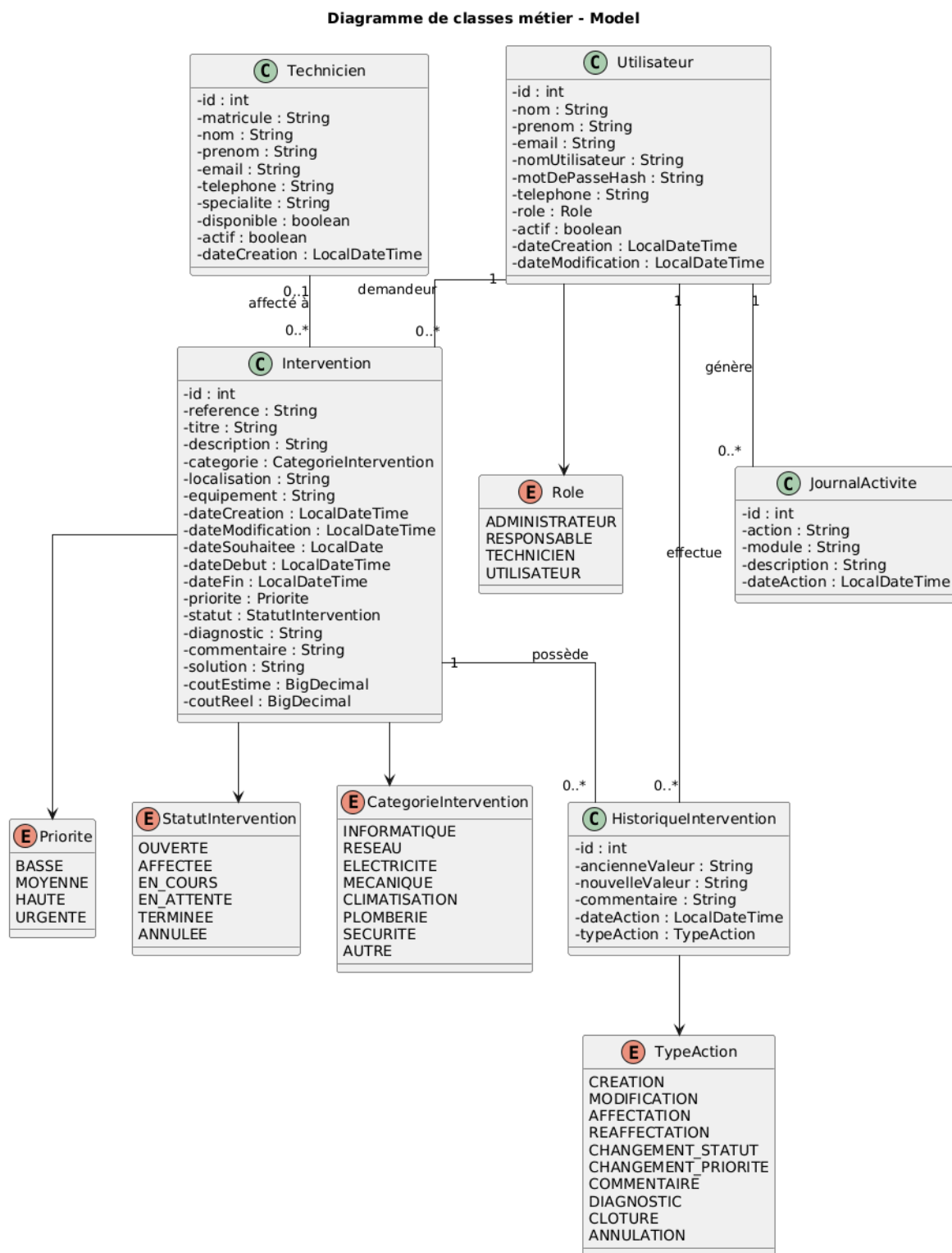
Figure 8 : Diagramme des classes métier
