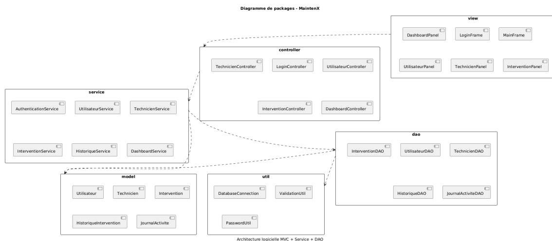
Figure 26 : Organisation des packages
