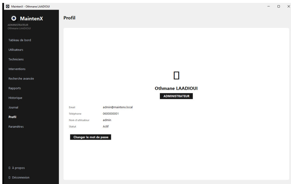
Figure 36 : Profil utilisateur
