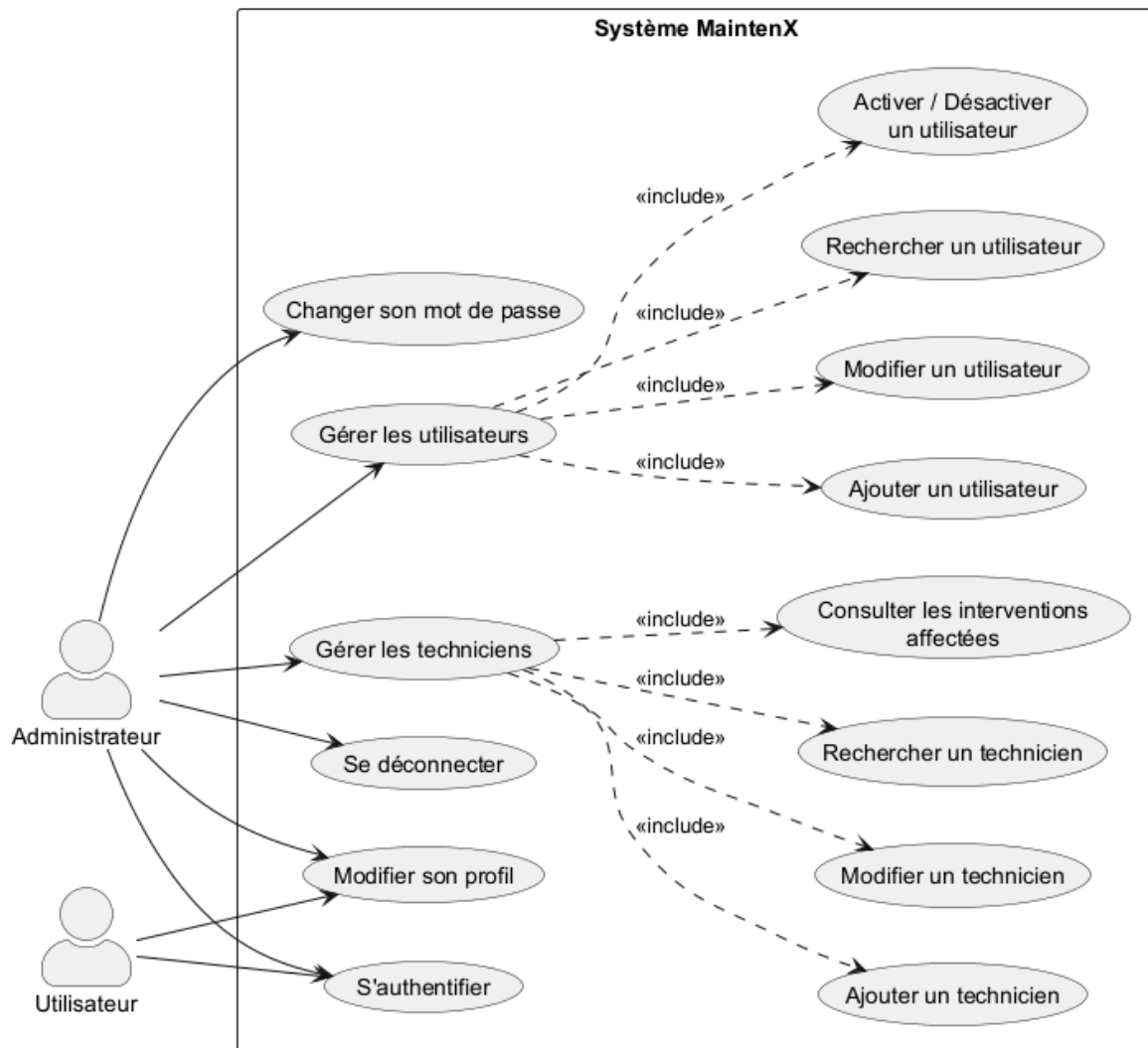
Partie 1/3 du diagramme global
