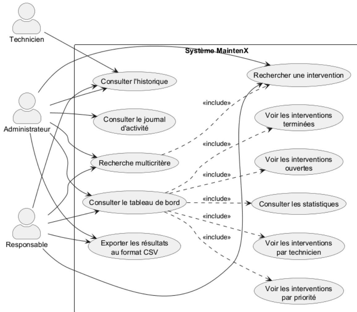
Partie 3/3 du diagramme global
