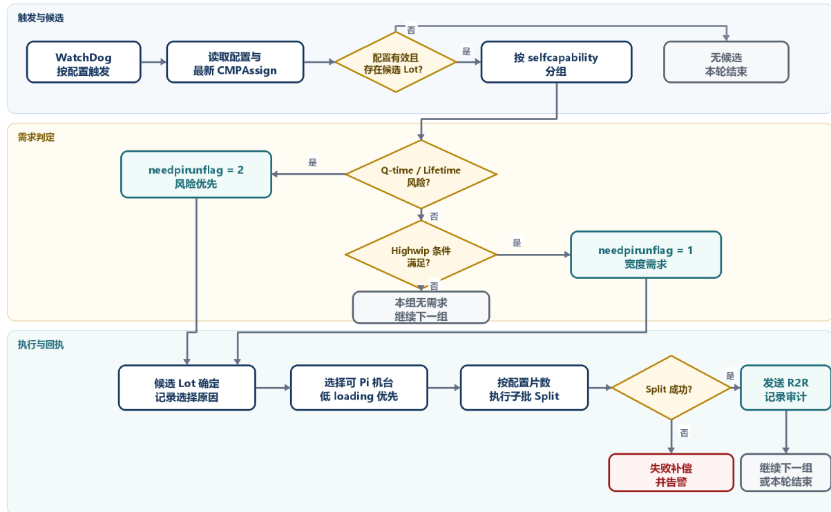
图 2 CMPAutoPirun 主决策流程
