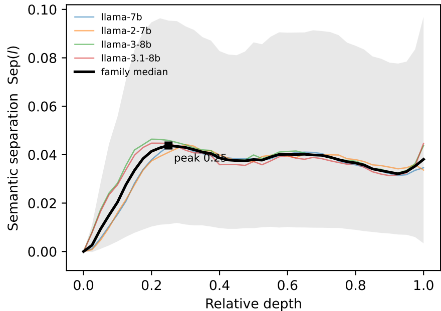
LLaMA family
