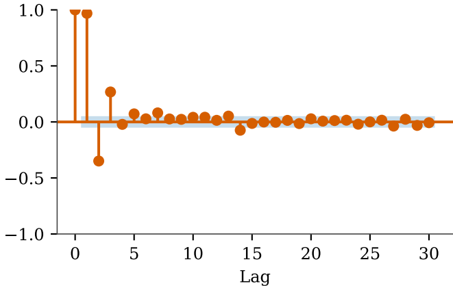
Swift Creek -- PACF
