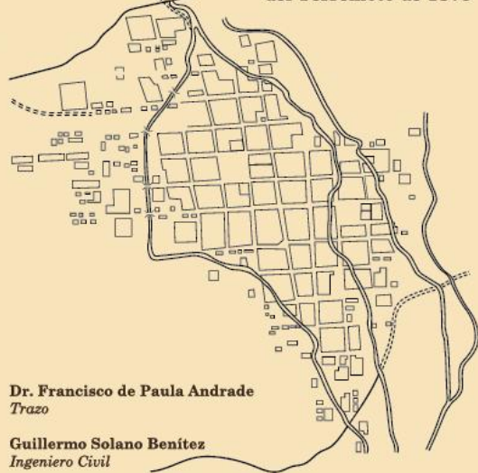
Traza de Cúcuta antes del Terremoto de 1875
