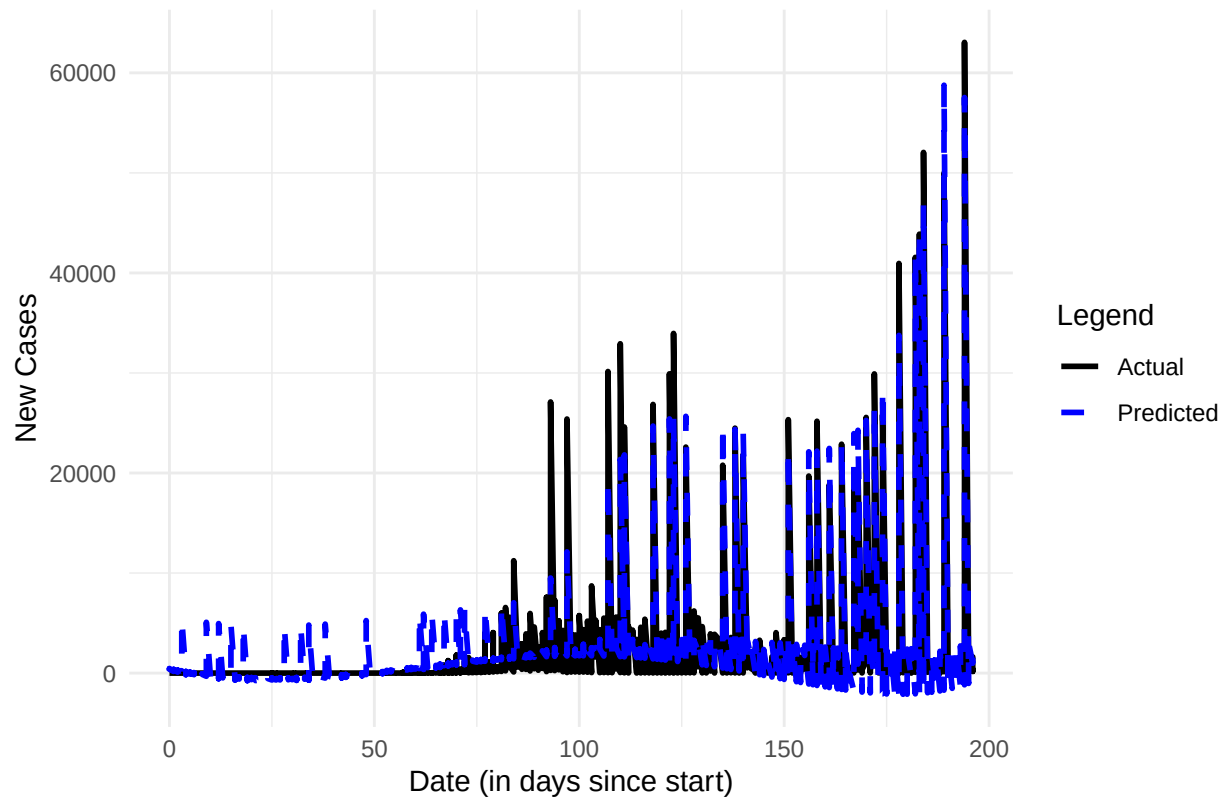
Actual vs Predicted New Cases (Test Set)
