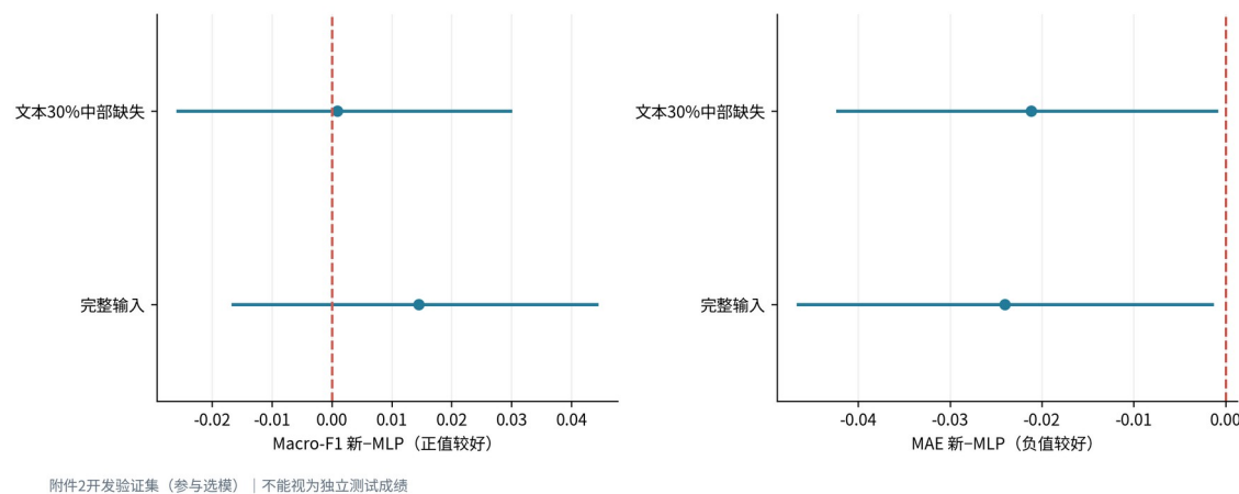
图 11 EMT-DLFR 相对 MLP 的配对差值及 95%分组 Bootstrap 区间
