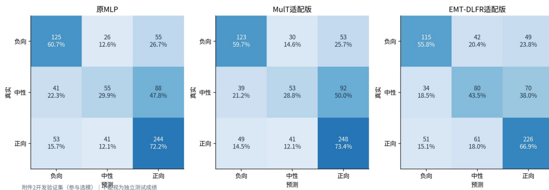
图9 MLP、Mult 与 EMT-DLFR 的逐类识别表现
