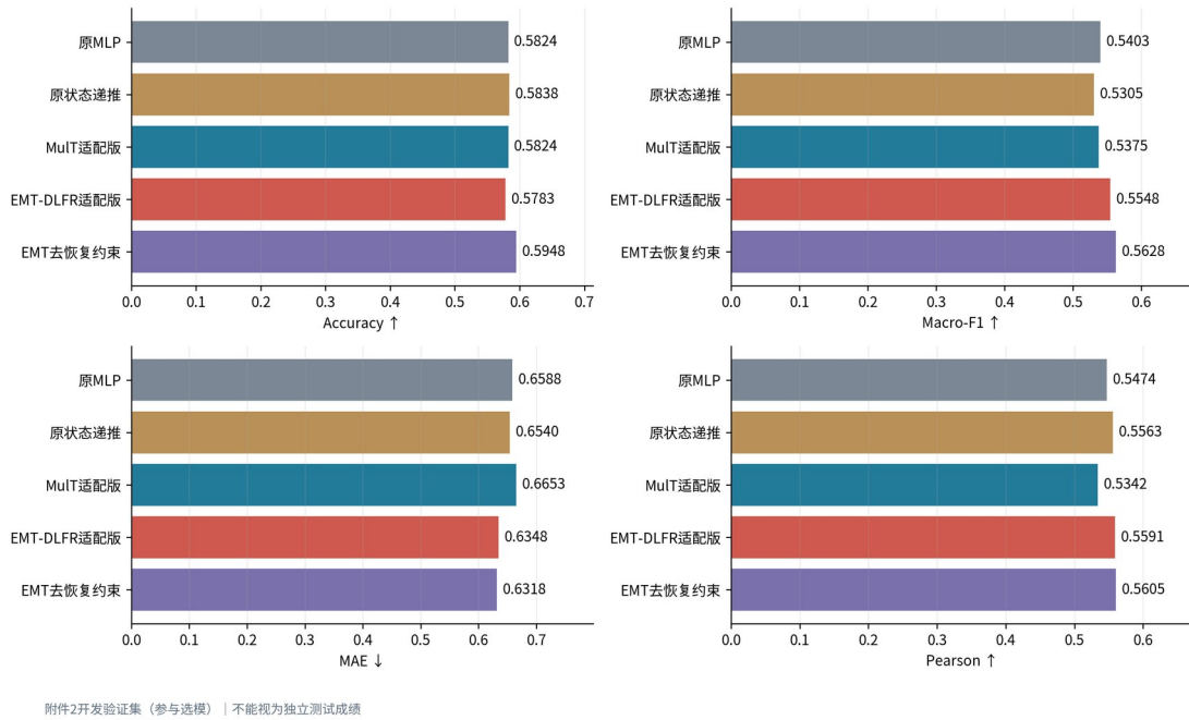
图4 未追加人工遮挡下的五种方法集成性能
