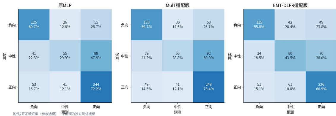
图 10 MLP、Mult 与 EMT-DLFR 的逐类识别表现
