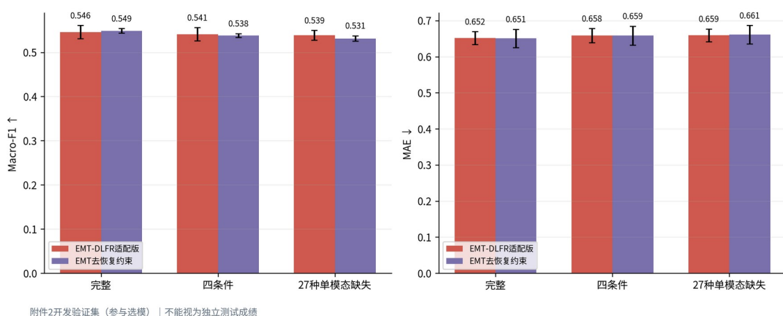
图9 两级恢复约束消融：保持相同的完整/缺失视图监督
