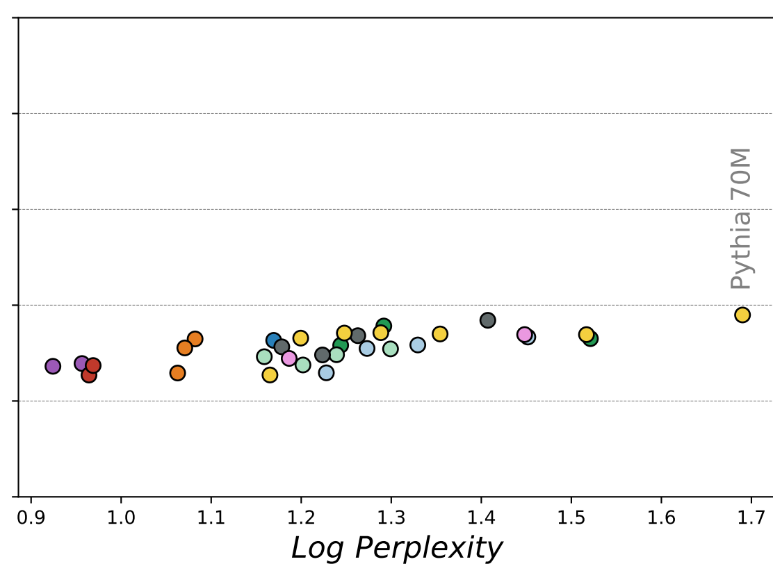
Passages
