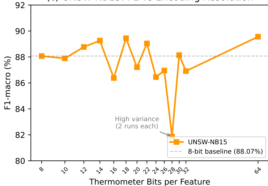
(c) UNSW-NB15: F1 vs Encoding Resolution
