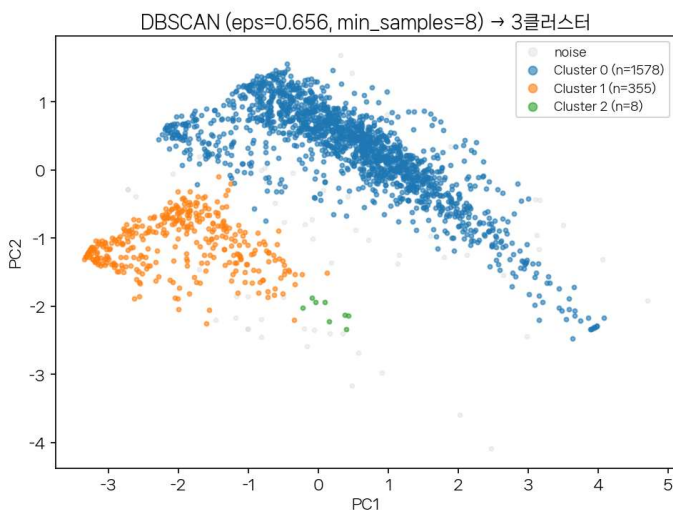
[그림 2] DBSCAN 보조 검증 결과. K-Means 후보군 380명 중 355명이 동일 밀집 군집에 포함됐다.
