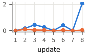
grad norm
