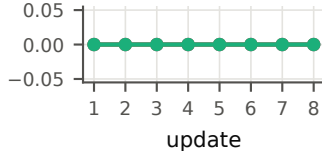
clip fraction
