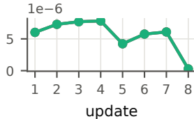
update KL(old||new)
