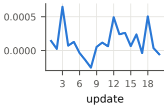
grad norm
