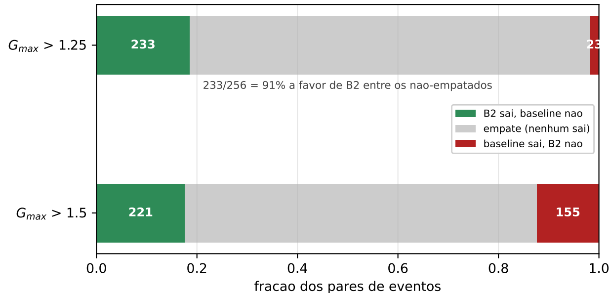
B) quem sai da brecha primeiro, no mesmo evento (proporcao; sem media, sem modelo)
