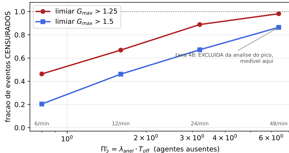
A) a brecha nao fecha antes do proximo evento (censura = medida direta de \Pi_2 )
