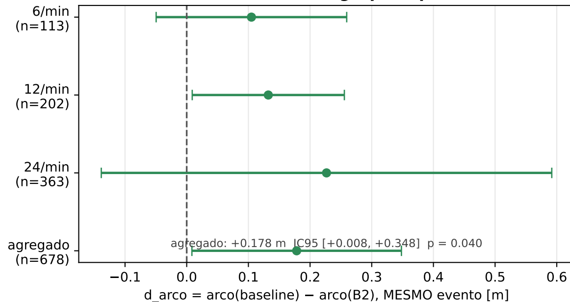
B) diferenca pareada por evento (media; barras = IC95 agrupado por rodada)
