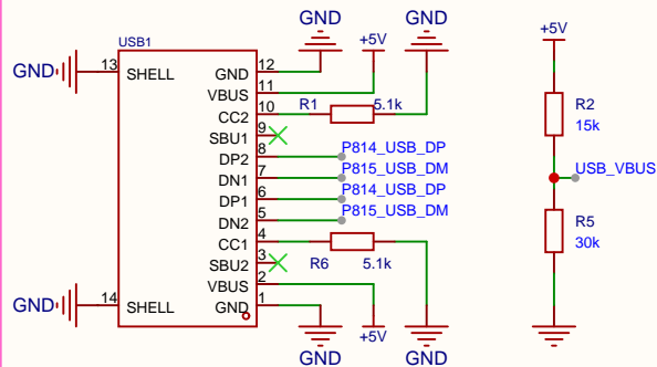
Type-C供电/下载
