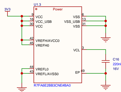
R7FA6E2BB3CNE_电源
