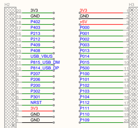
拓展接口
