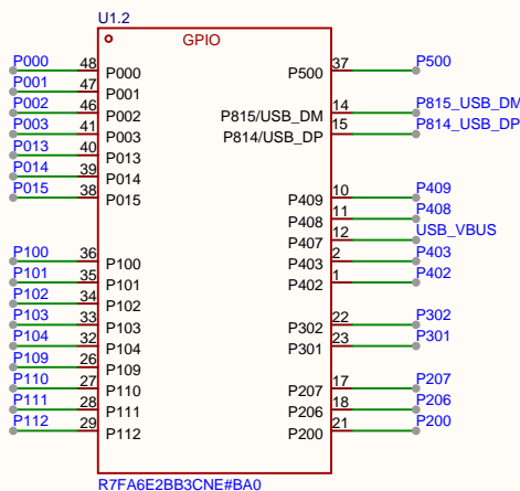
R7FA6E2BB3CNE_IO
