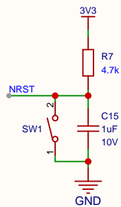
复位电路
