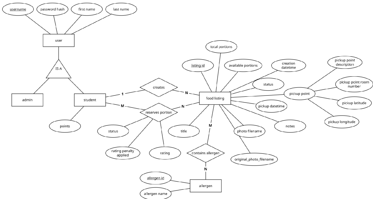
Εικόνα 1 — Διάγραμμα Οντοτήτων-Συσχετίσεων (ER Diagram).
