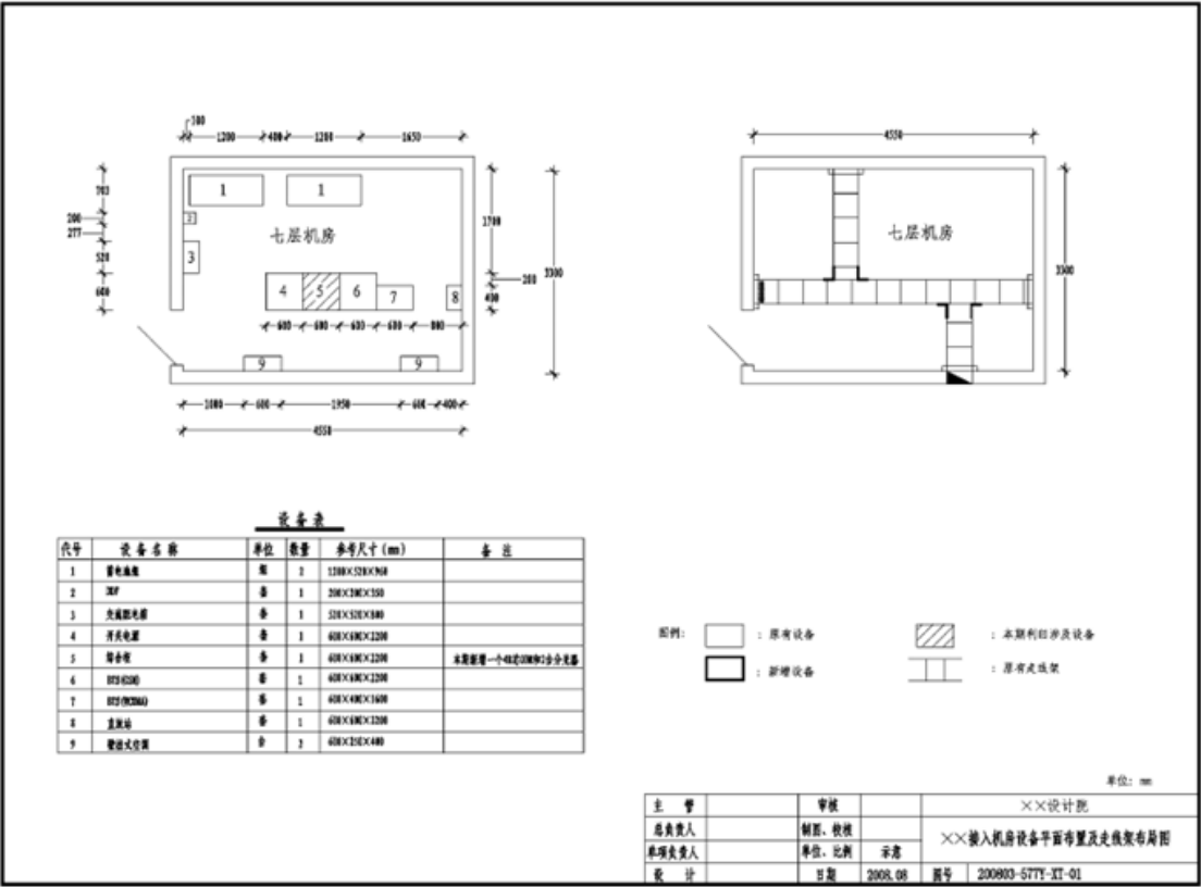
图4-15 接入机房设备平面布置图
