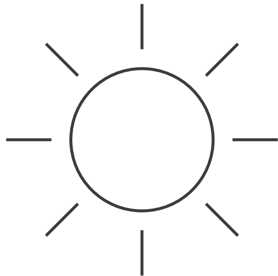
Sun
